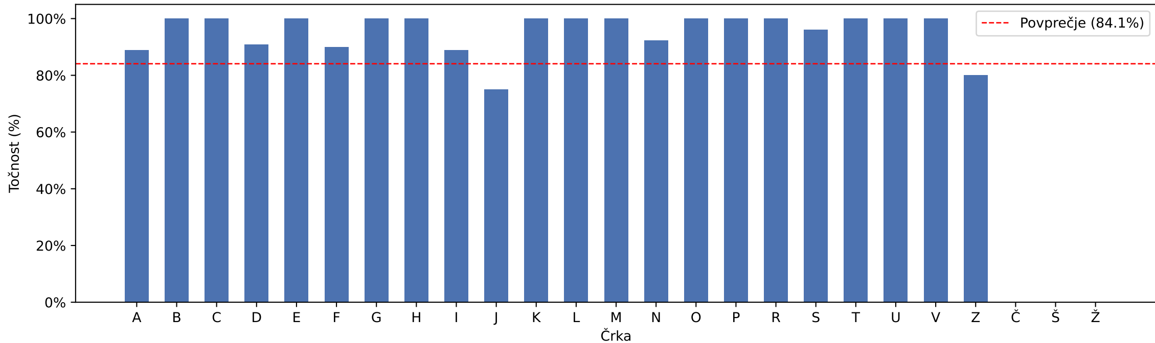
Točnost po razredih — Model A (EMNIST original)
